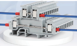
Двухуровневая клемная колодка
